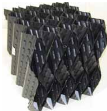
(Altezza/height mm 130)
