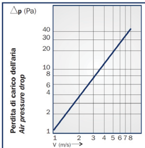
(Altezza/height mm 130)
